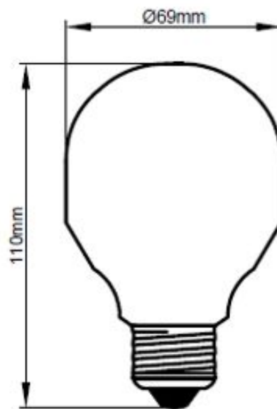
A60-PS60-E27(IEC60630)
