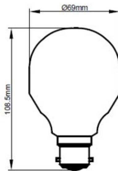
A60-PS60-B22(IEC60630)
